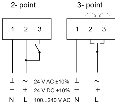
Schema elettrico
